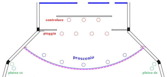
DISPOSIZIONE FARI
